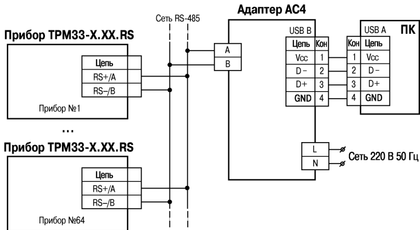
Рисунок В.5 – Схема подключения TPM33-X.X.RS к адаптеру сети AC4
